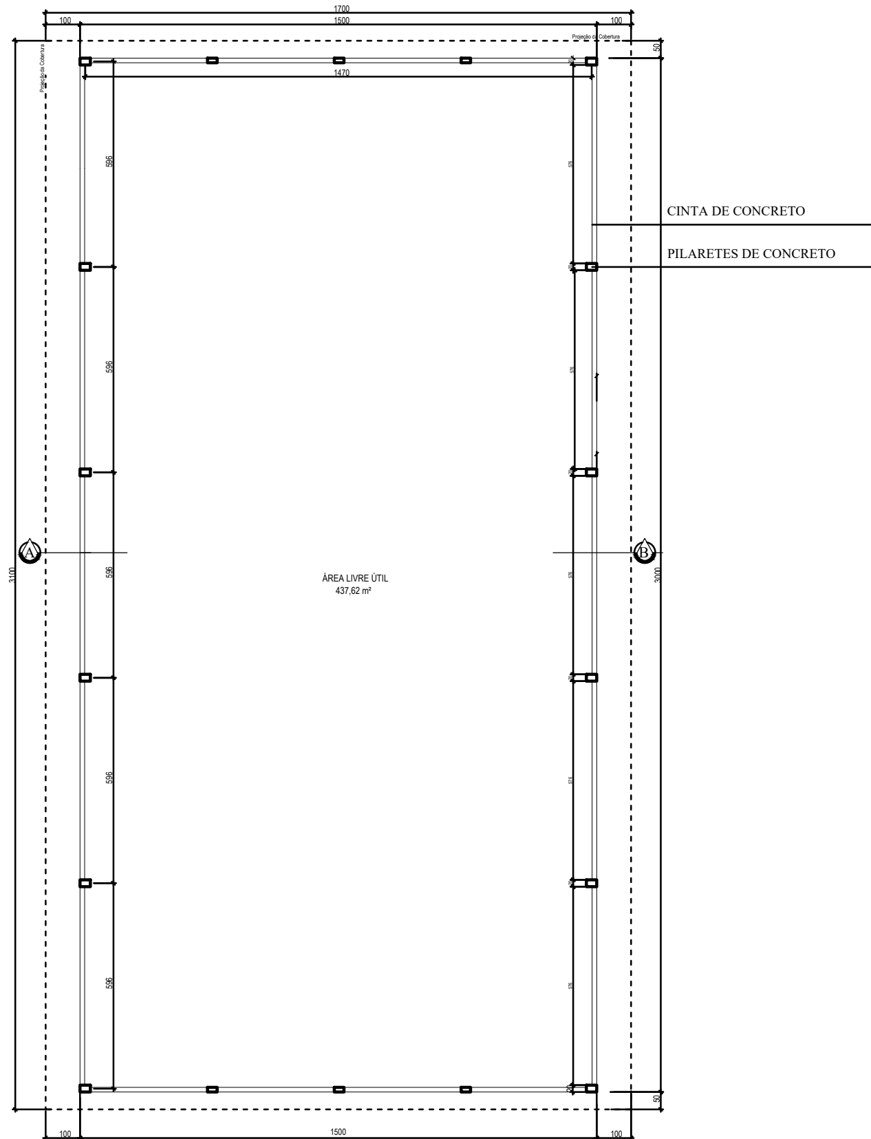
○ PL. BAIXA GALPÃO ESC. 1/75
