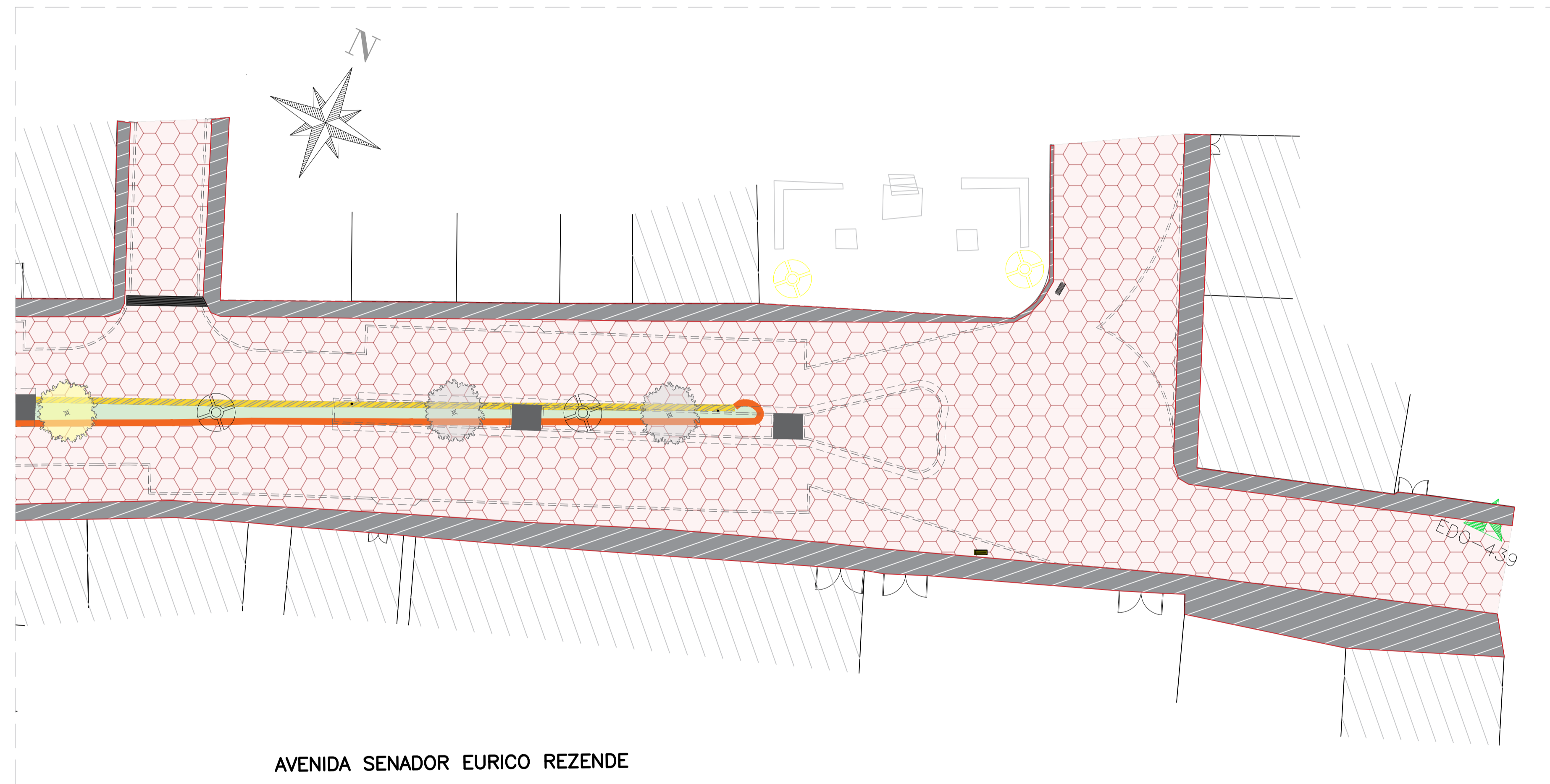
PLANTA DE DEMOLIÇÃO - 03 ESC.:1/250
